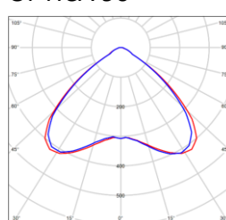
ÓPTICA 90°
