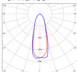
ÓPTICA 30°
