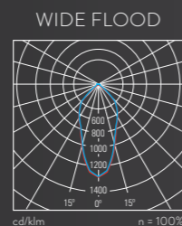
— C0 - C180 — C90 - C270 Curvas fotométricas correspondentes a 4000K.
